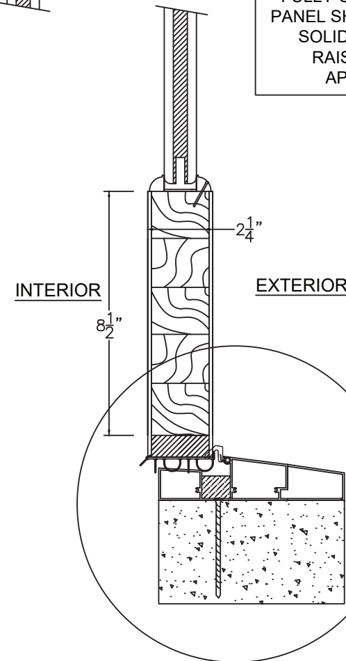
B INFILL DOOR SECTION
