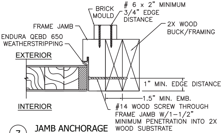
7 JAMB ANCHORAGE
